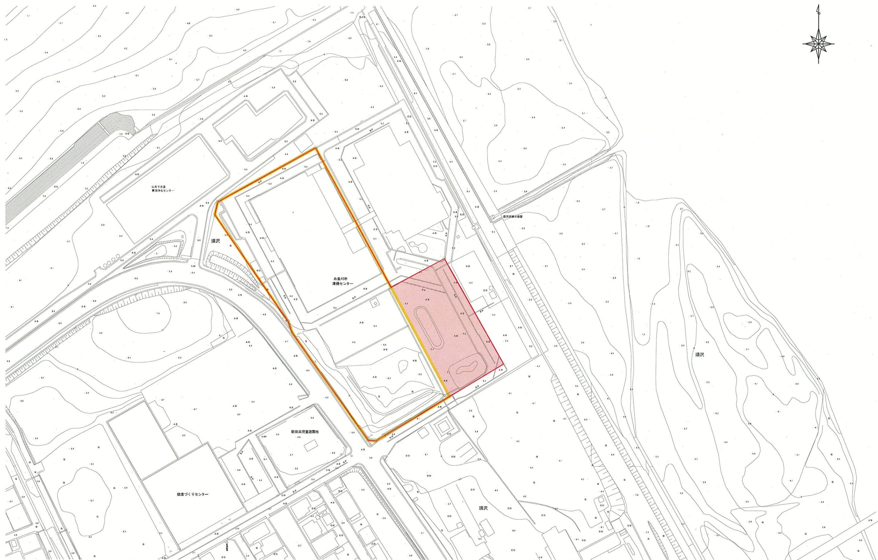
糸魚川都市計画ごみ焼却場計画図 A1 : S=1/600 A3 : S=1/1200
